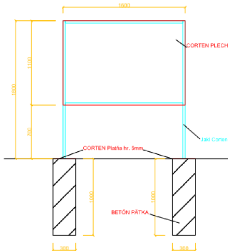
pohľad predný
